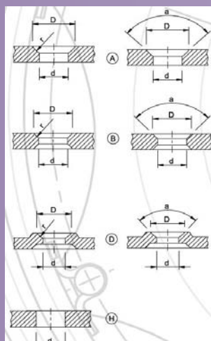
Pallokartiotyypit Kartioreikätyypit
